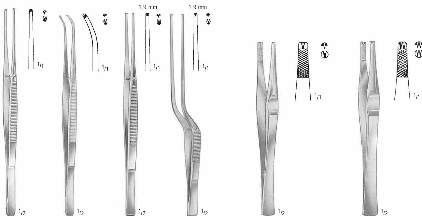
TAYLOR 1:2 AB 150/17 17,5 cm/7" TAYLOR 1:2 AB 151/17 17,5 cm/7" TAYLOR 1:2 AB 152/17 17,5 cm/7" TAYLOR 1:2 AB 153/17 17,5 cm/7" LANE 1:2 AB 156/14 AB 156/20 14,5 cm/5¾" 20,0 cm/8" LANE 2:3 AB 158/14 AB 158/20
